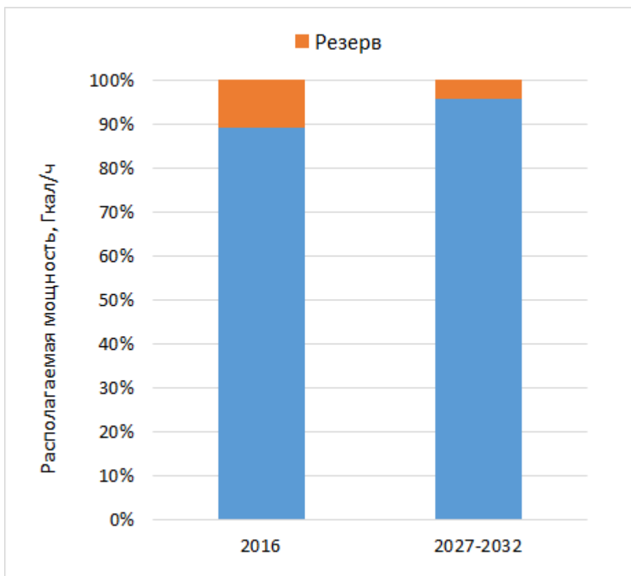
Рисунок 2.3. Балансы тепловой мощности и перспективной тепловой нагрузки котельной №36 д. Сяськелево
