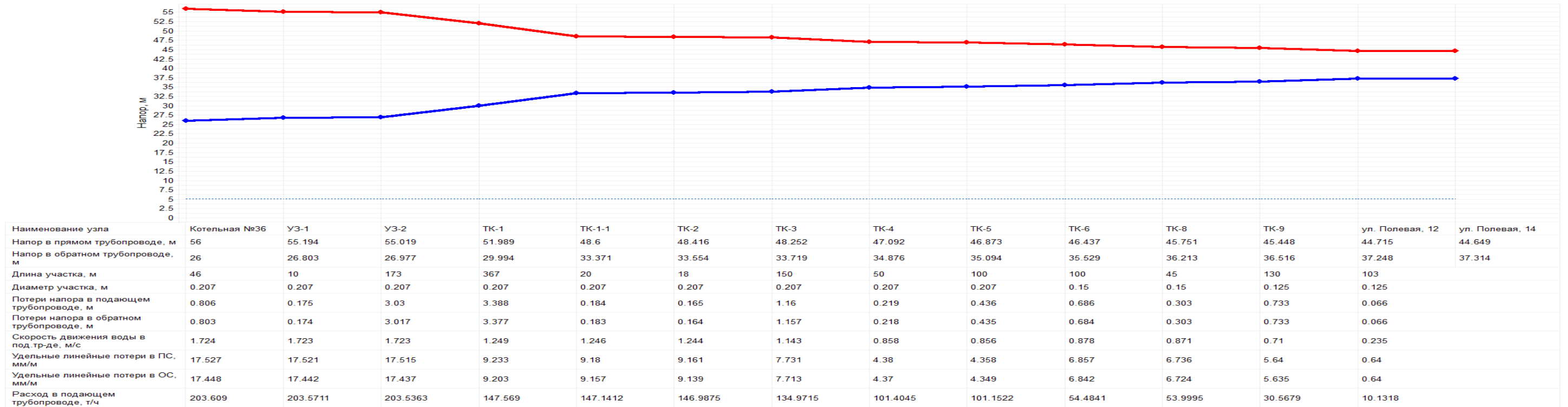
Пьезометрический график контура отопления от котельной №36 д. Сяськелево до ул. Полевая д. 14
