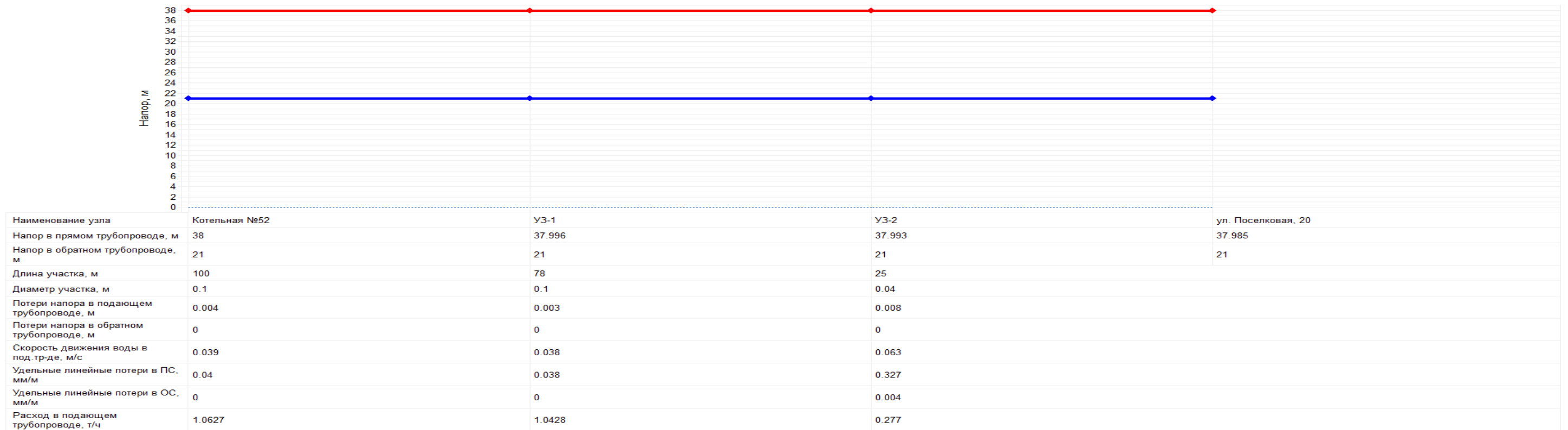
Пьезометрический график контура ГВС от котельной №52 д. Жабино до ул. Поселковая д. 20
